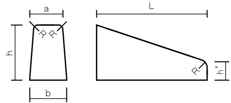
(両面 B・C)直端部
